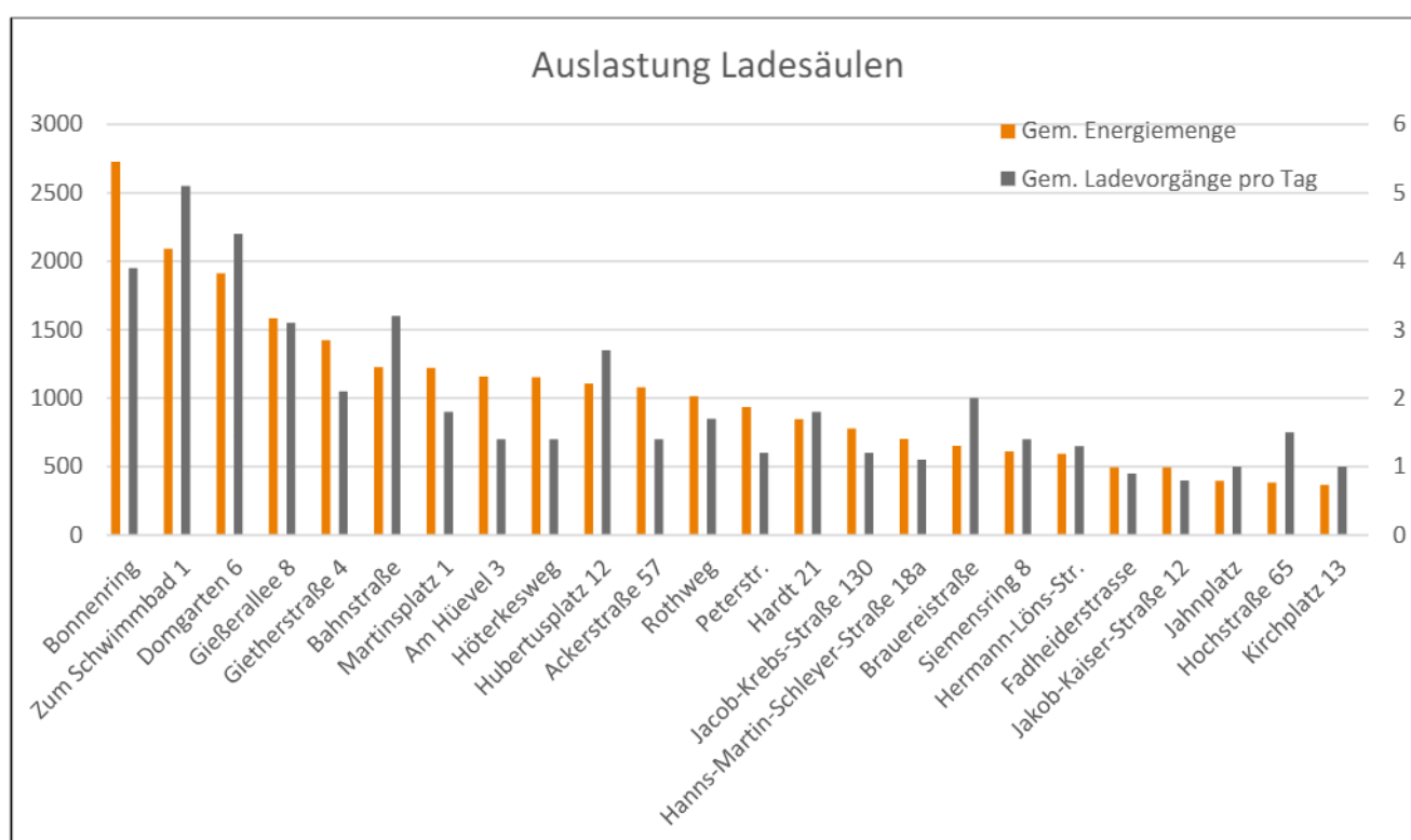
Abbildung 5: Energiemenge und Ladevorgänge pro Tag
